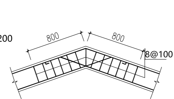
坡屋面板折角 折梁剖面加筋示意
