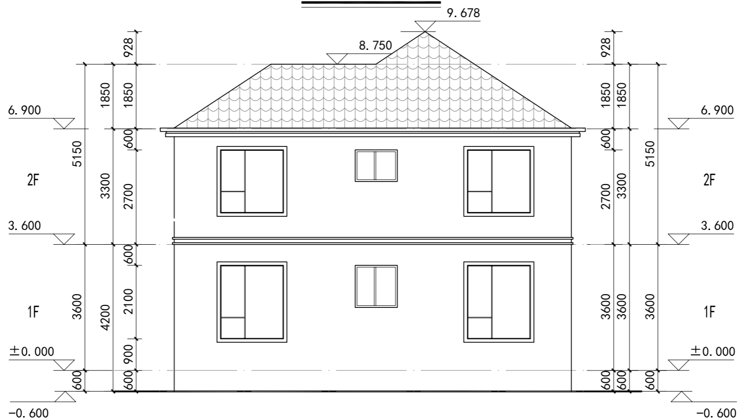
正立面图 1:100
