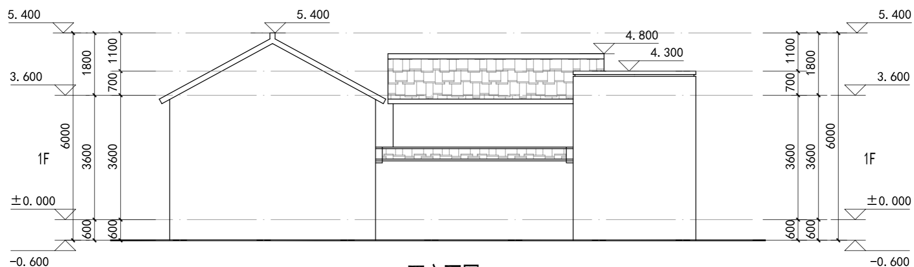
西立面图 1:100
