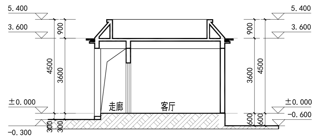
1-1剖面图 1:100
