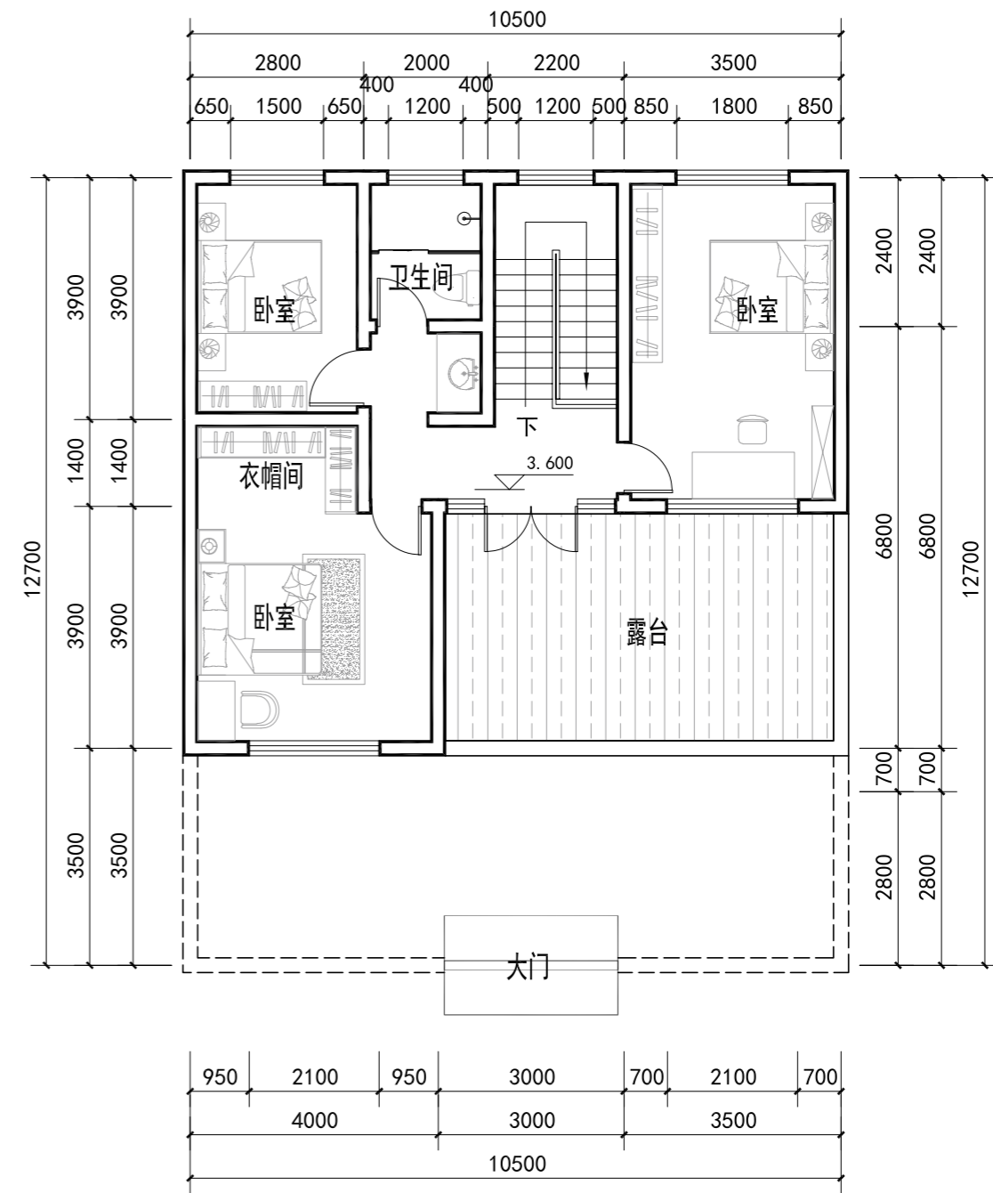
二层平面图 1:100 建筑面积: 76.04m 2
