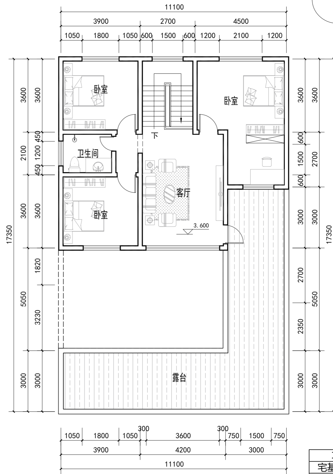
二层平面图 1:100 建筑面积: 99.18m 2
