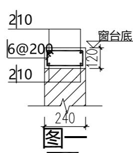
注:沿外墙窗台底通长设置
