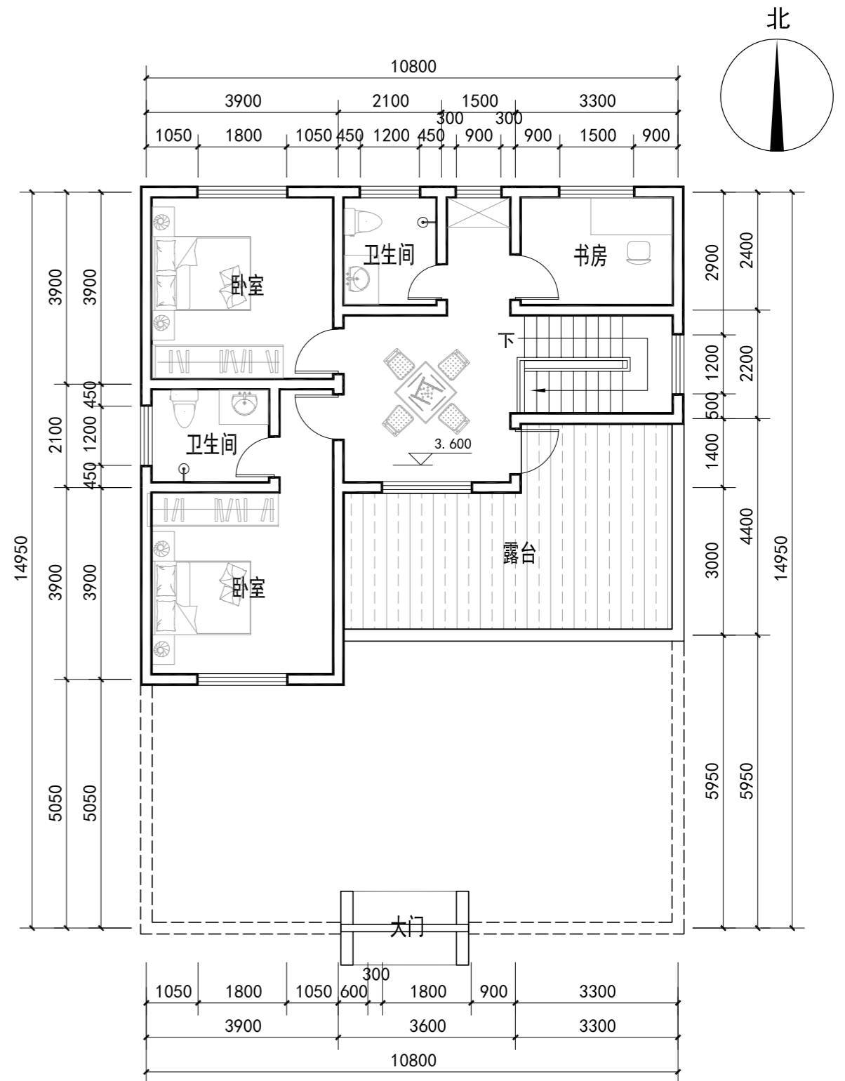
二层平面图 1:100 建筑面积: 80.42m 2
