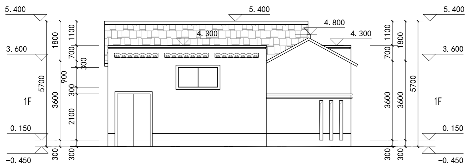
正立面图 1:100
