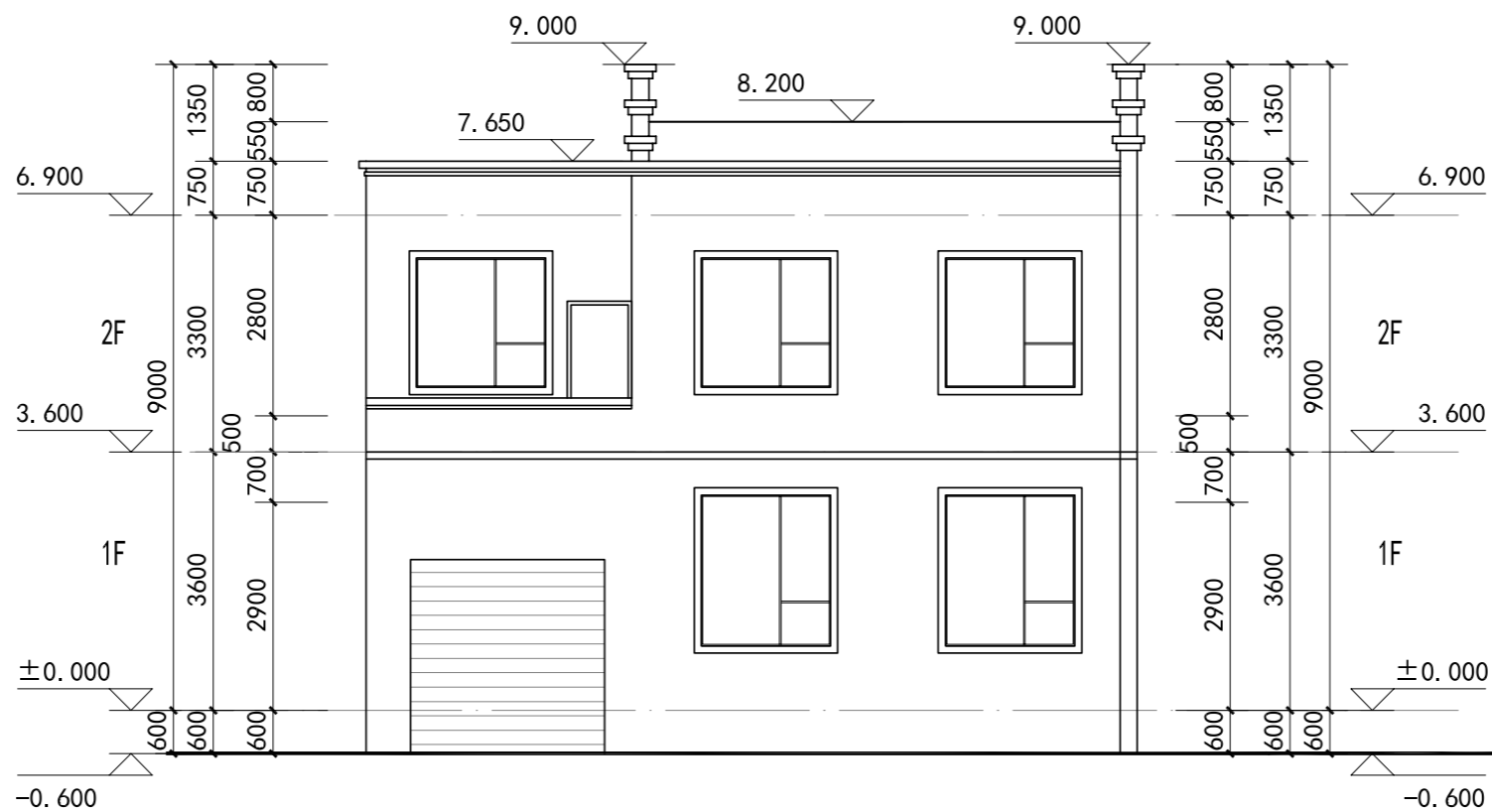
背立面图 1:100
