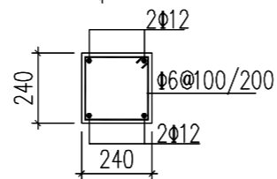
GZ1详图
