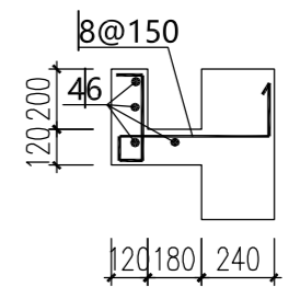
檐口详图 平面位置详见建施图
