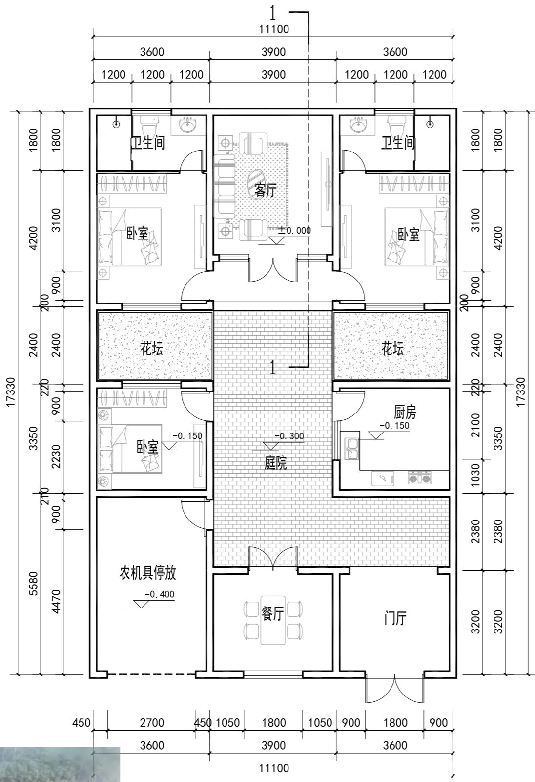
一层平面图 1:100 建筑面积: 127.69m 2
