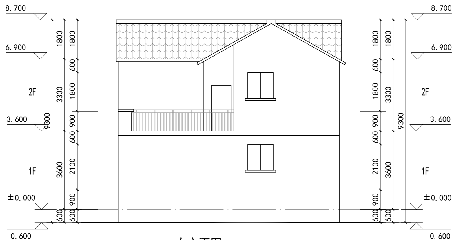
东立面图 1:100
