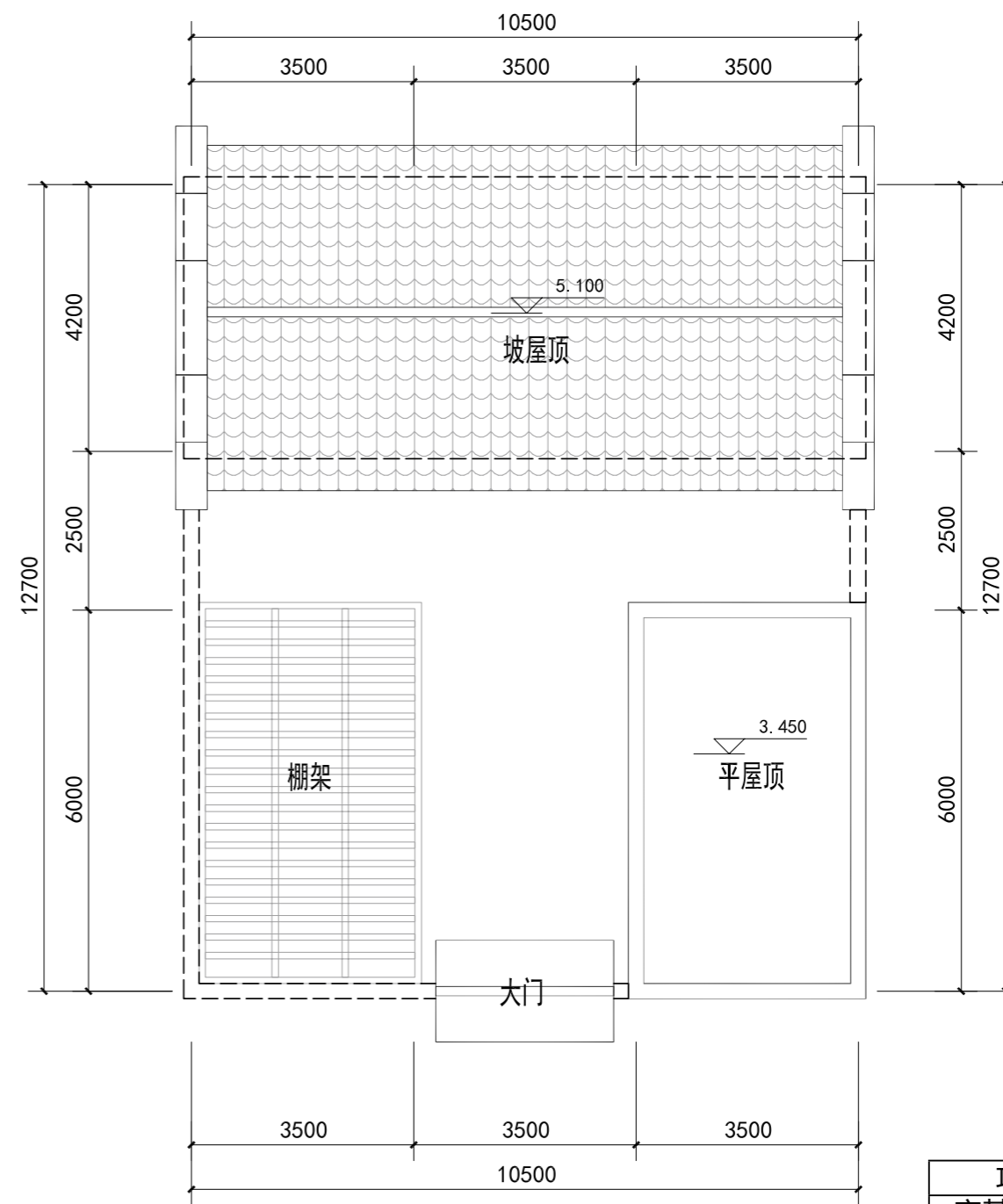
屋顶层平面图 1:100
